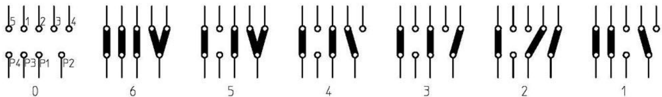
Schaltschema bei Rechtsdrehung
